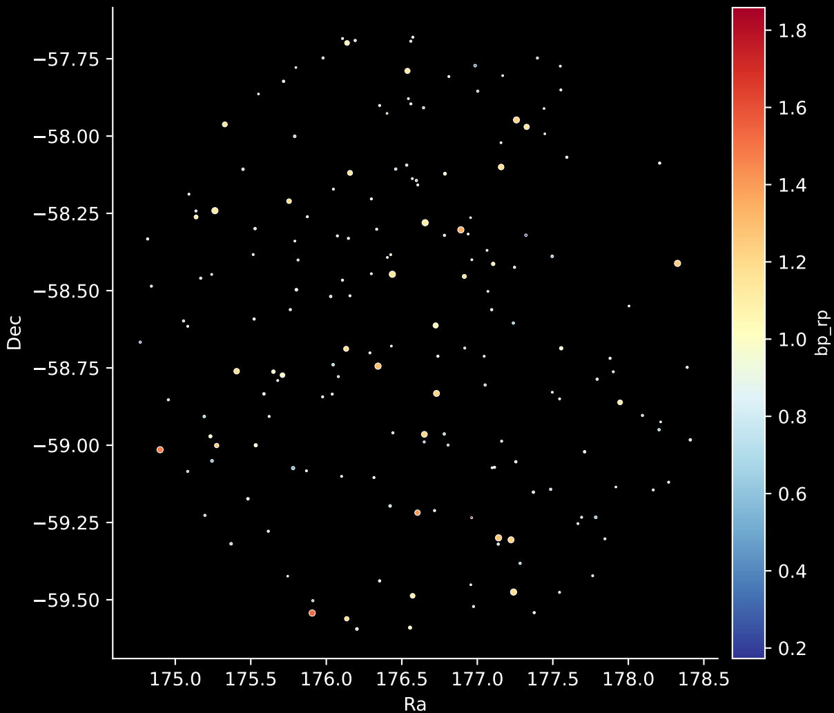
GALAH DR4 Field: [7183] Stars: 178
