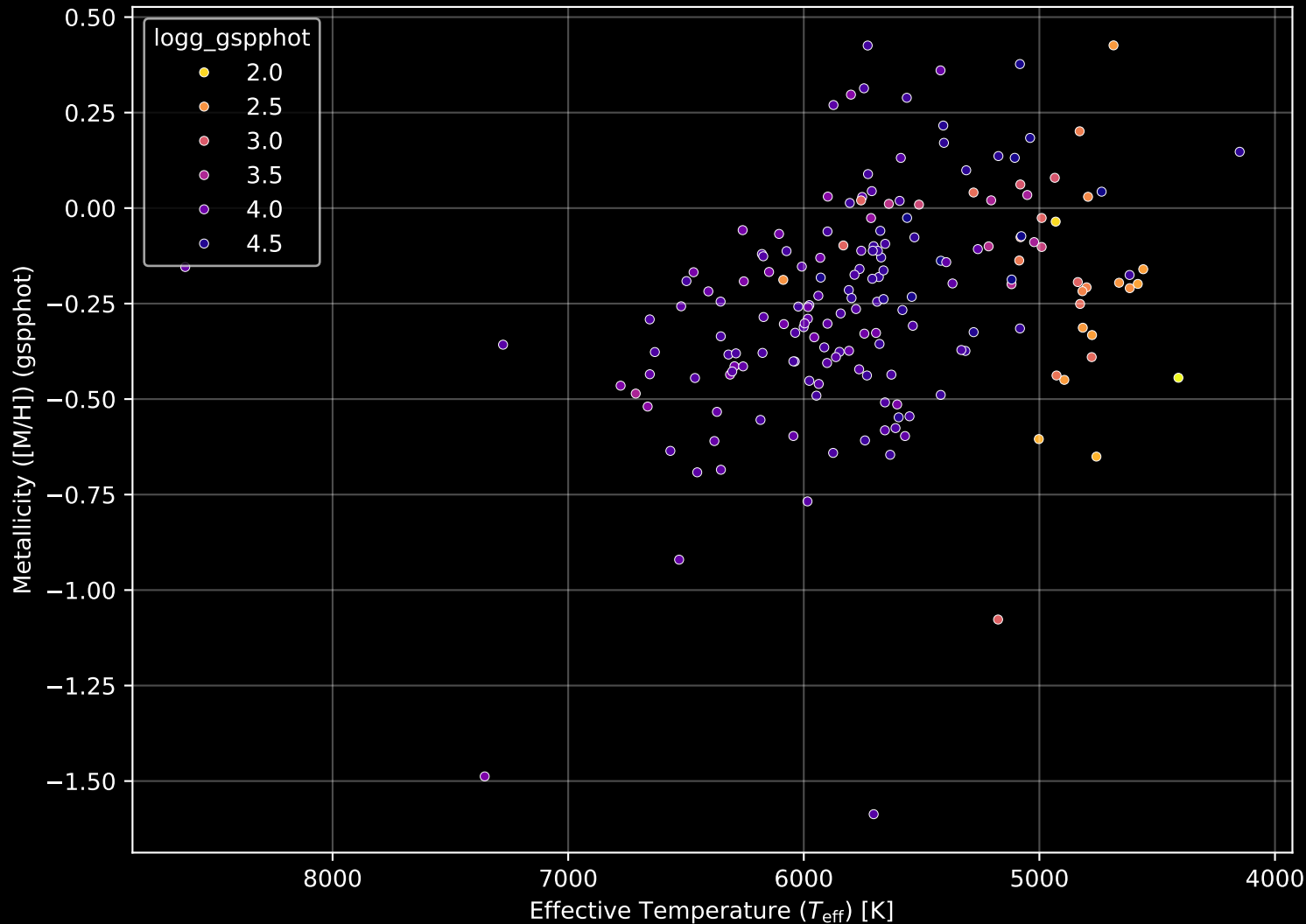
GALAH DR4 Field: [7183] Stellar Population Parameters (n= 178)
