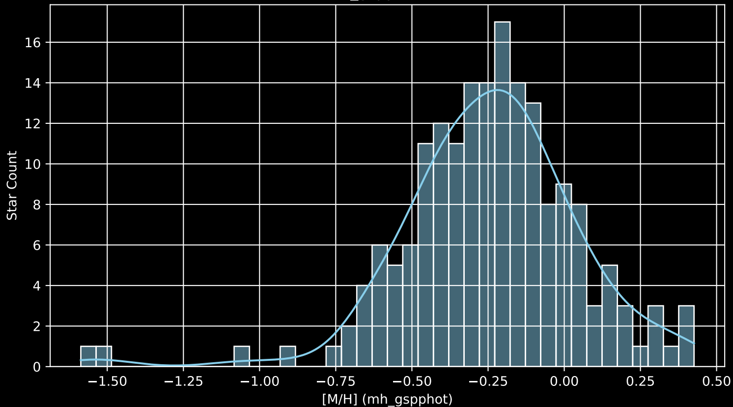
GALAH DR4 Field: [7183] [M/H] (mh_gspphot) (n= 178)
