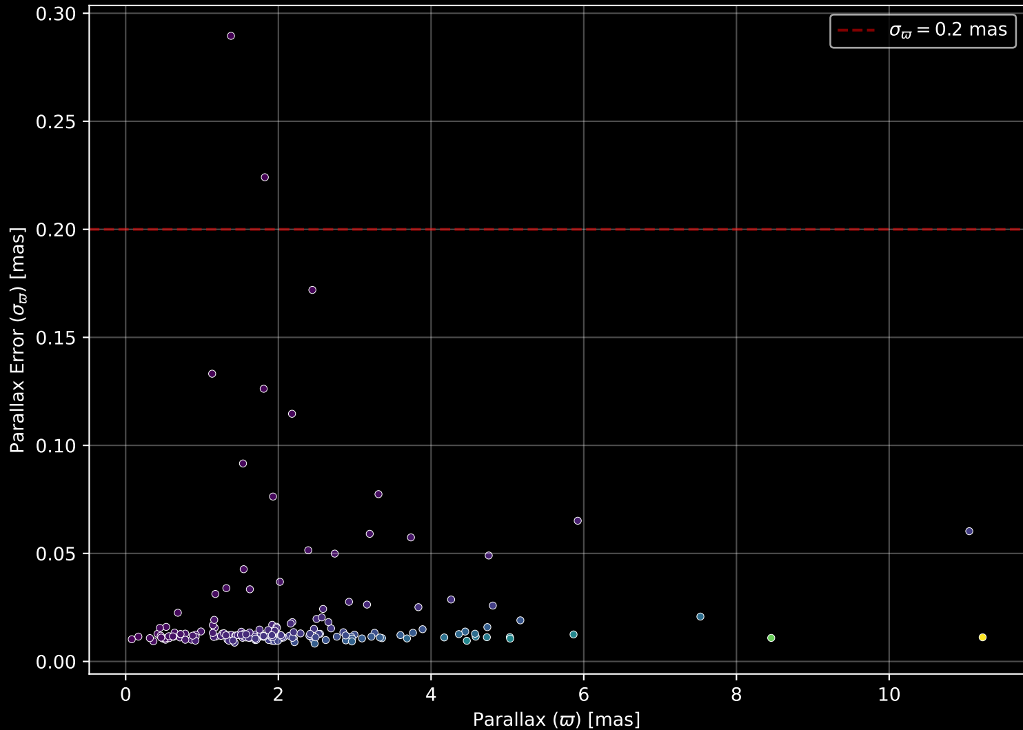
GALAH DR4 Field: [7183] Parallax Quality (n= 178)
